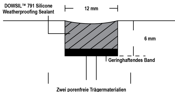
Abbildung 2: Flache Fuge
